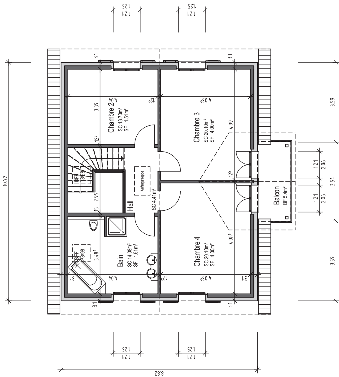
Etage 1:100
